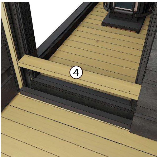
10. Placez la planche de seuil ( 4 ) entre le sauna et le vestiaire
