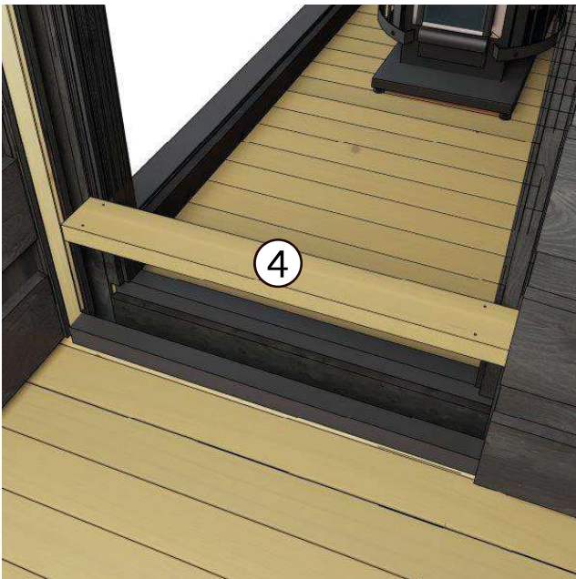
10. Plaats de drempel ( 4 ) tussen de sauna en de kleedkamer
