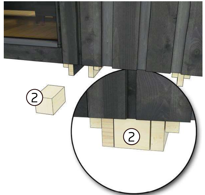
7. Placera utfyllnadsbiten ( 2 ) mellan transportstöden.
