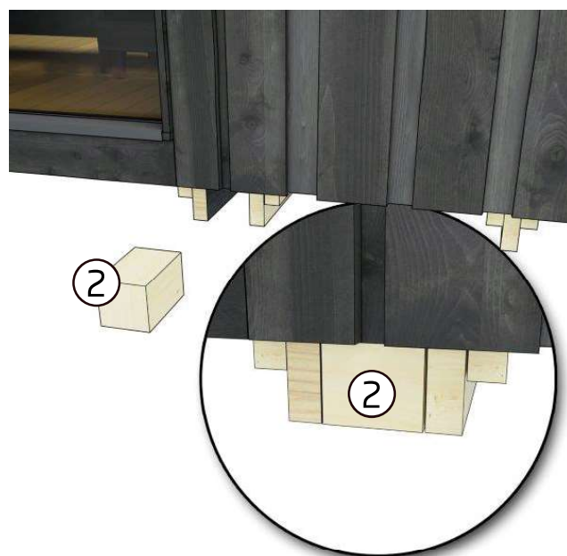
7. Plaats het opvulelement (2) tussen de transportbeugels.
