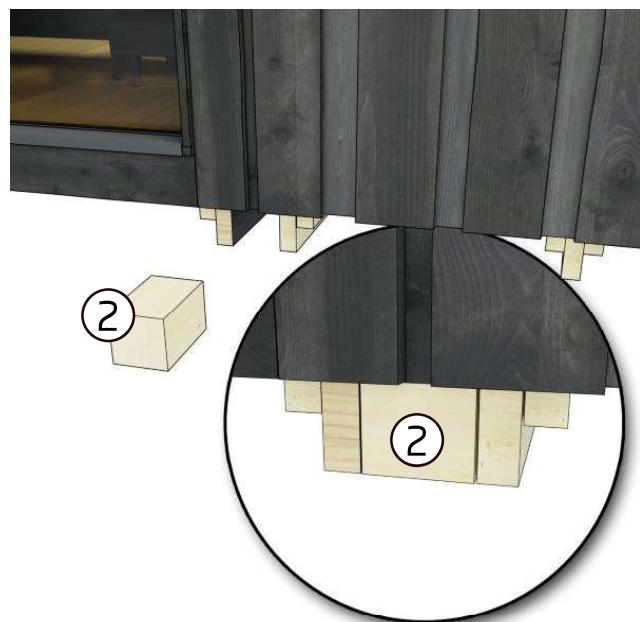
7. Laita täytepala ( 2 ) saunan ja pukuhuoneen kuljetustukien väliin.
