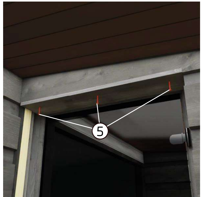
12. Kiinnitä Smyygilauta lyhyt ( 6 ) saunan ja pukuhuoneen oviaukon ylös. Smyygilauta tulee päin saunan oven karmeja. Smyygilauta kiinnitetään kolmella ruuvilla ( 5 ). Smyygilaudassa on reiät valmiina.
